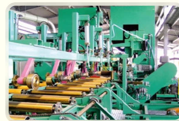
自動仕分け装置・定規連動ロールユニット装置付(オプション)
